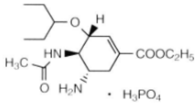
Oseltamivir phosphate
