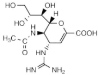
Zanamivir
